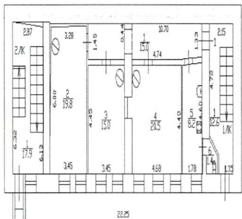
План 1 этажа
