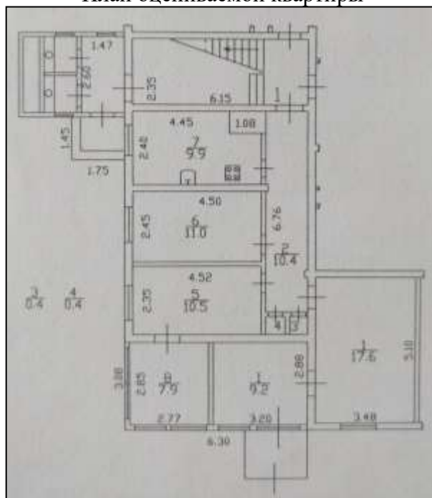
План оцениваемой квартиры
