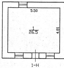
План 1 этажа h = 3.00
