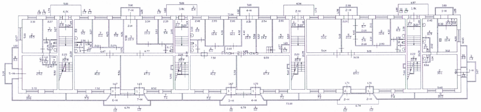
План 1 этажа
