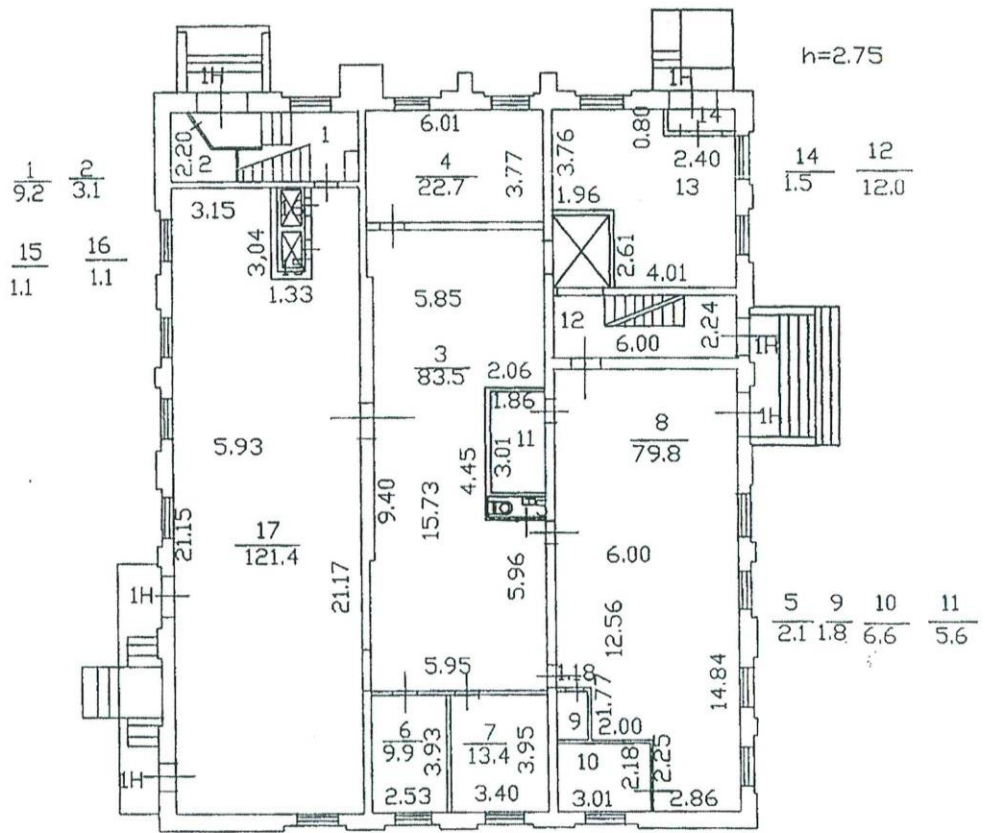
План 1 этажа
