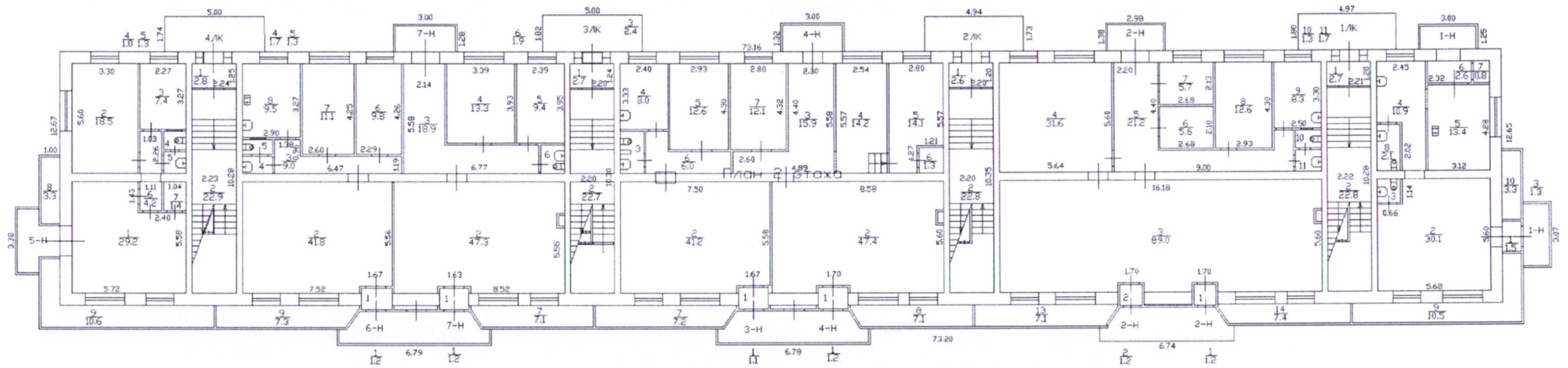
План 1 этажа
