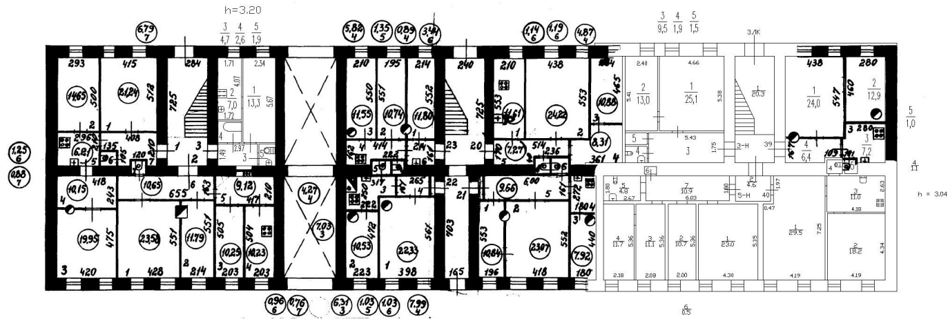
План 1 и цокольного этажей
