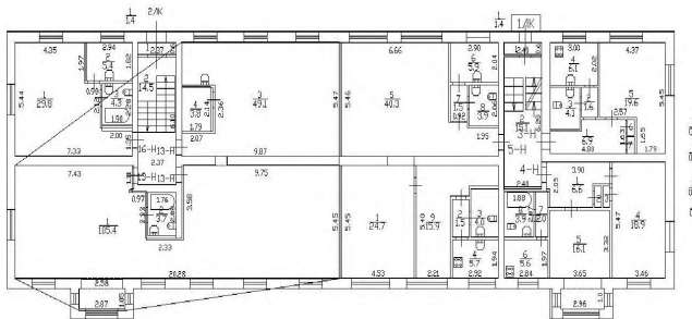
ПЛАН 1 ЭТАЖА
