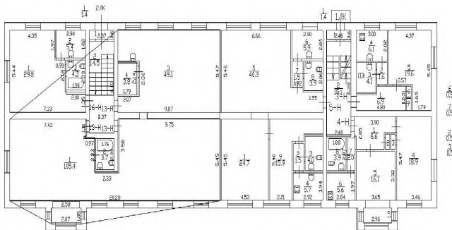
ПЛАН 1 ЭТАЖА
