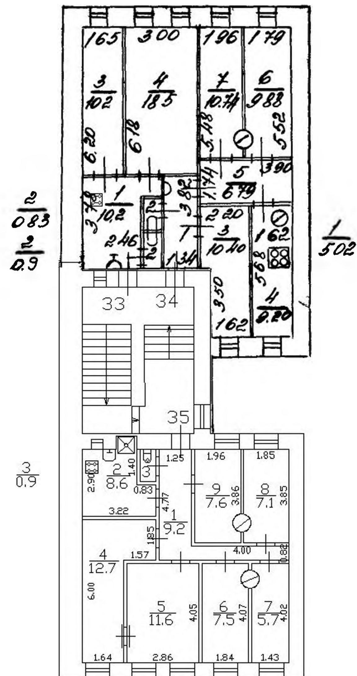
План 3 этажа
