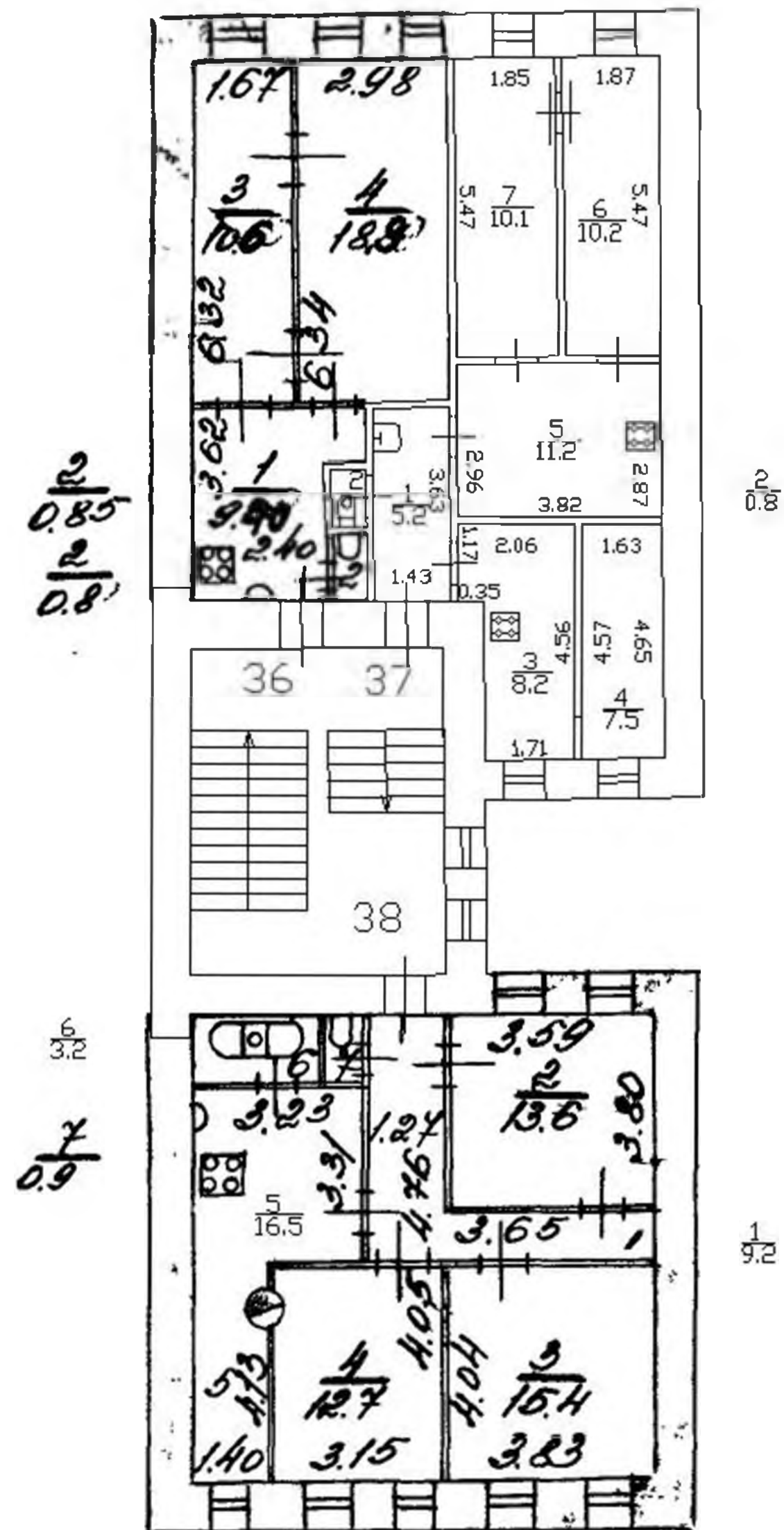
План 4 этажа
