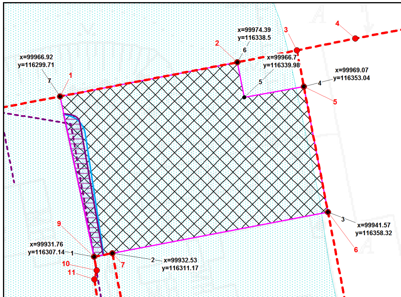
Схема расположения земельного участка в окружении смежно расположенных земельных участков (ситуационный план), 1:1200
