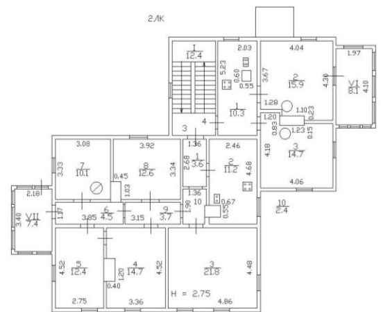
Рисунок 3. План 2-го этажа.
