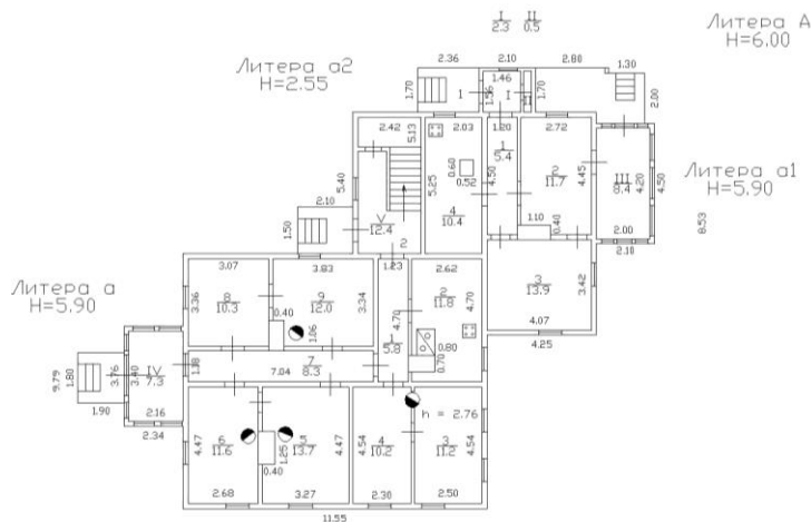
Рисунок 2. План 1-го этажа.
