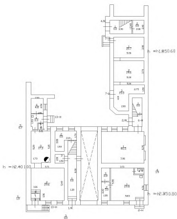
План подвала и цокольного этажа
