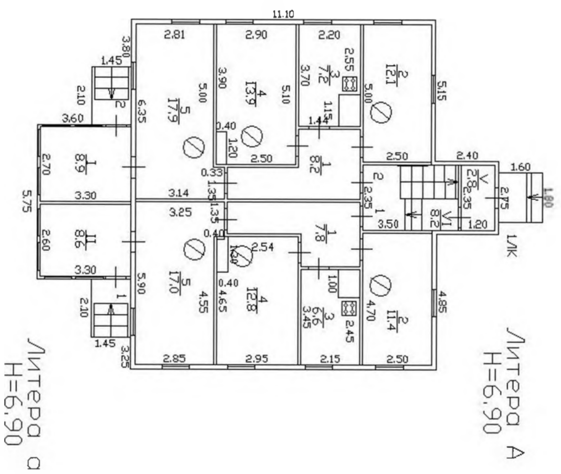
План 1 этажа
