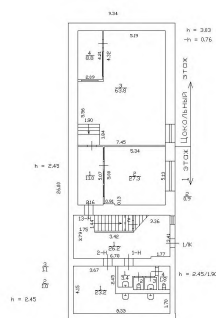
План цокольного - 1 этажа
