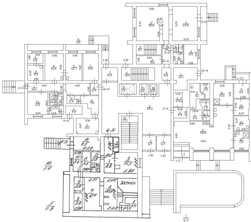
План 1 этажа h=2,55
