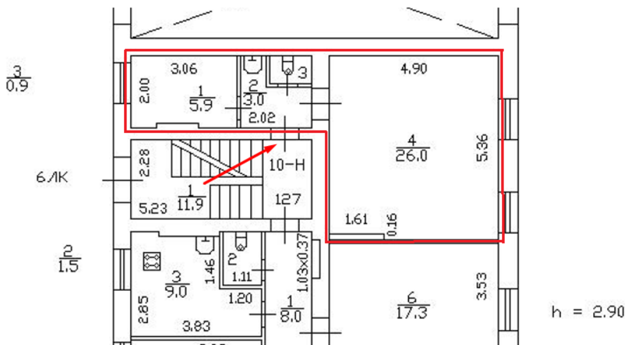
План помещения
