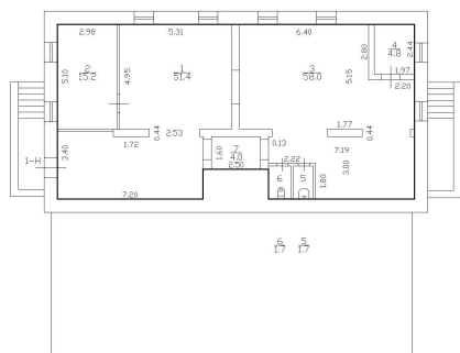
План цокольного этажа
