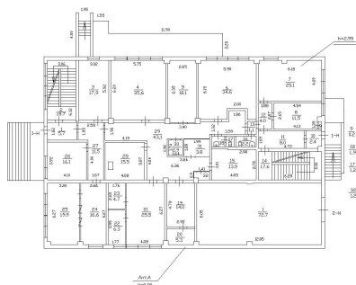
План 1 этажа
