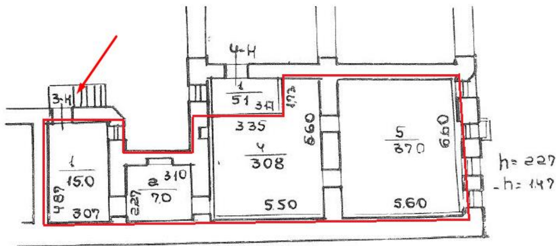
План помещения
