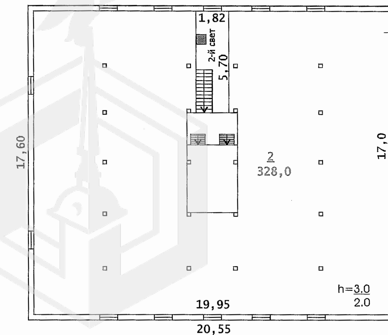
План 2 этажа
