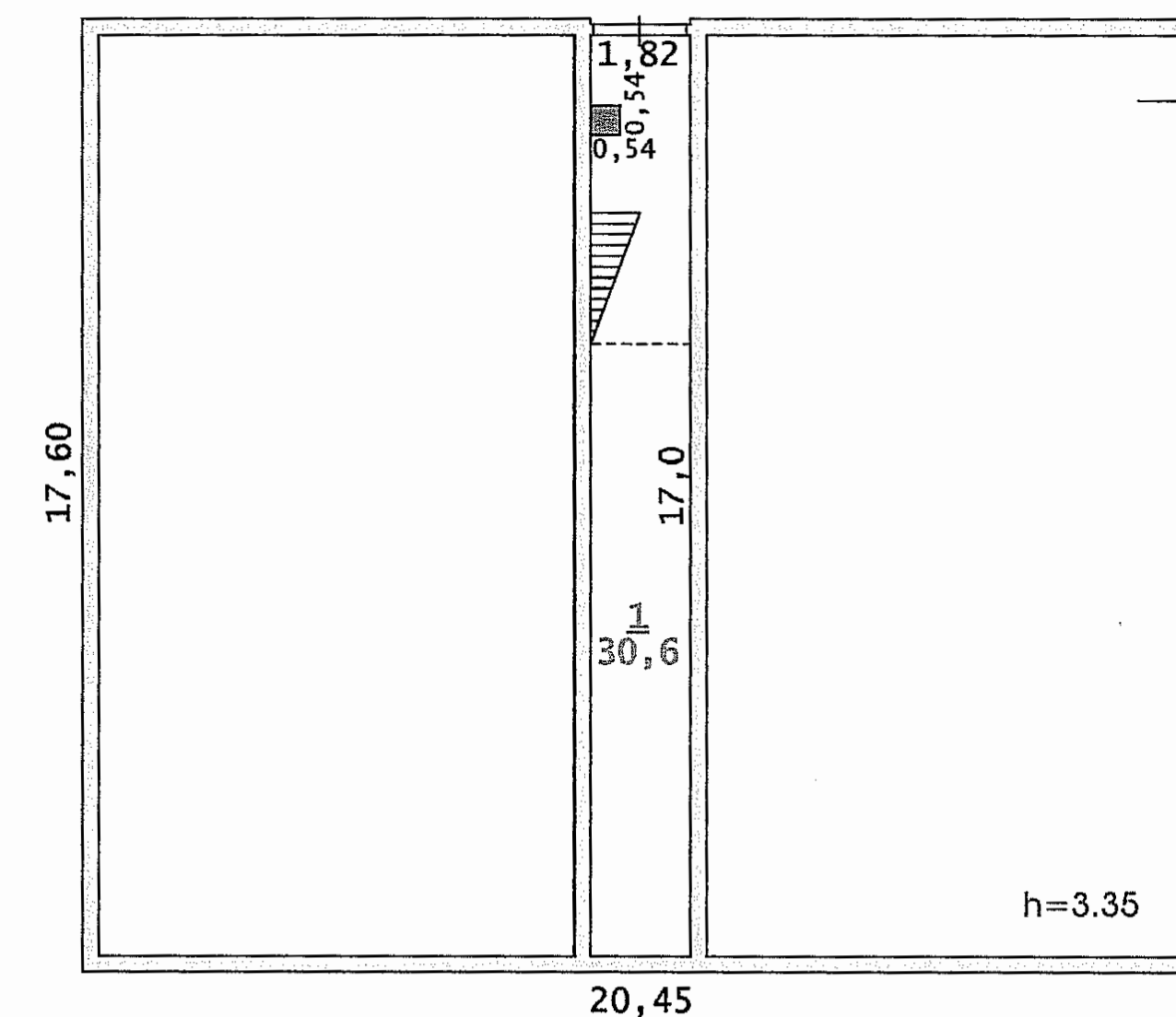
План 1 этажа
