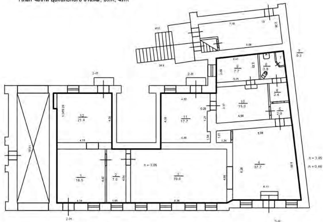
План части цокольного этажа, 3ЛК, 4ЛК
