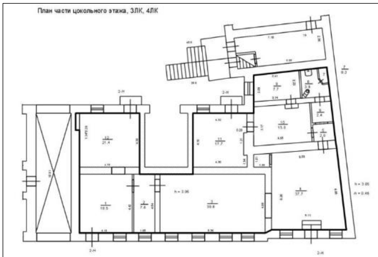
Рис. 3. Расположение помещения на плане цокольного этажа
