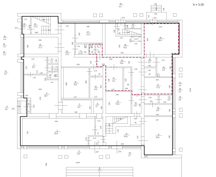
План 1 этажа
