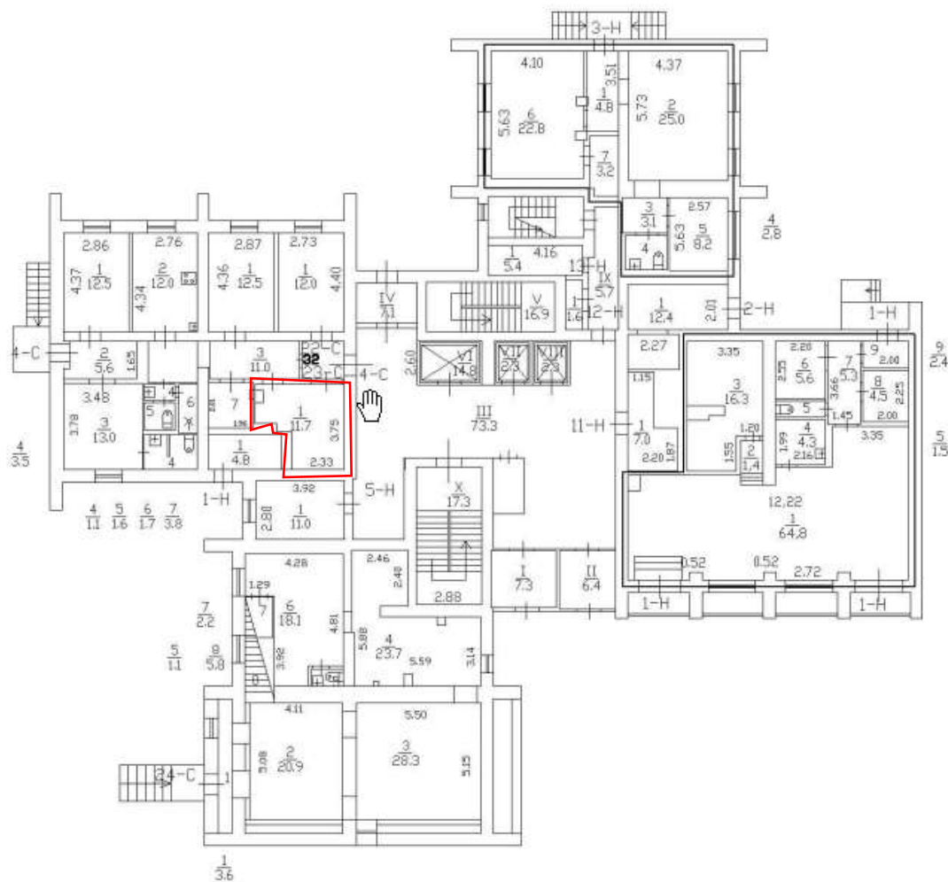
План 1 этажа h = 2.50
