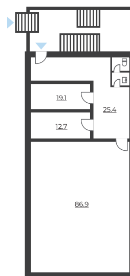
ПЛАН 1 ЭТАЖА ПОМ. 5-Н — 140,4 кв.м
