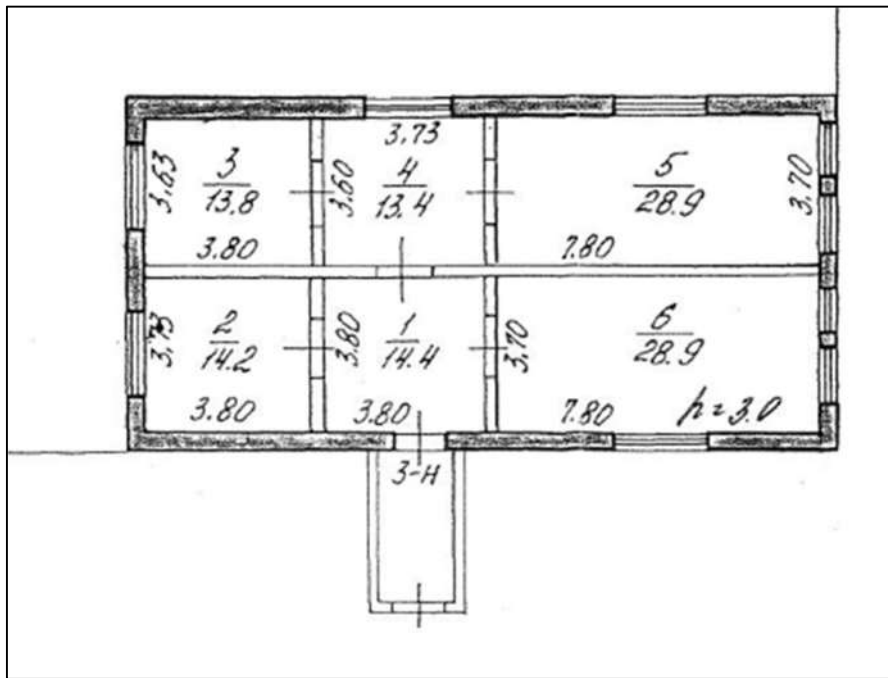
Рисунок 14. План 2 этажа здания литера Б
