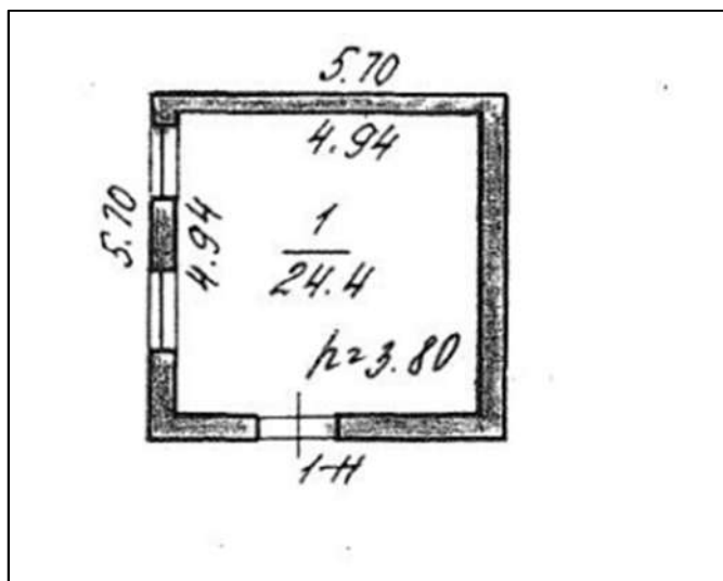
Рисунок 16. План 1 этажа здания литера Д
