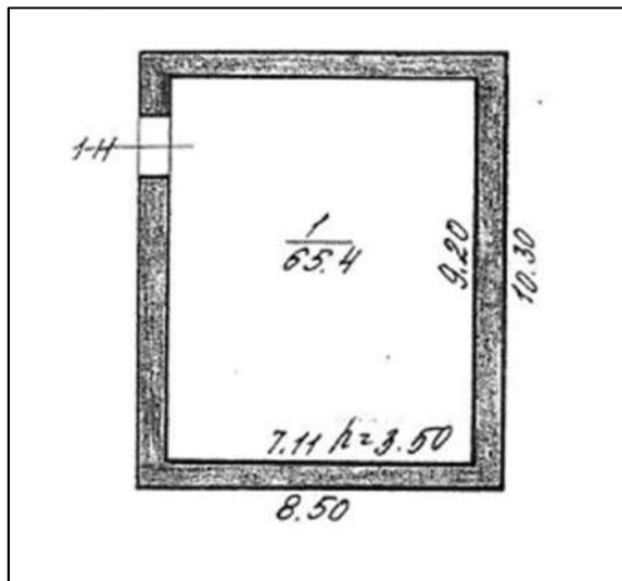
Рисунок 15. План 1 этажа здания литера В
