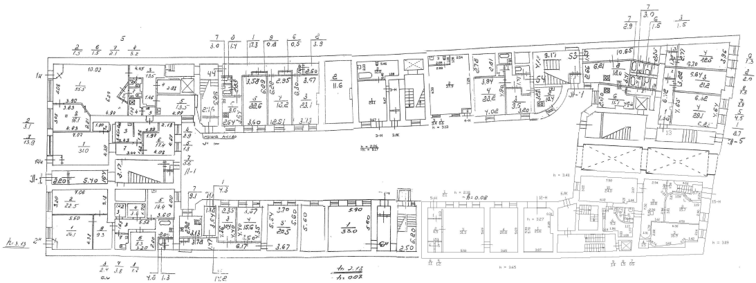
План цокольного - 1 этажа
