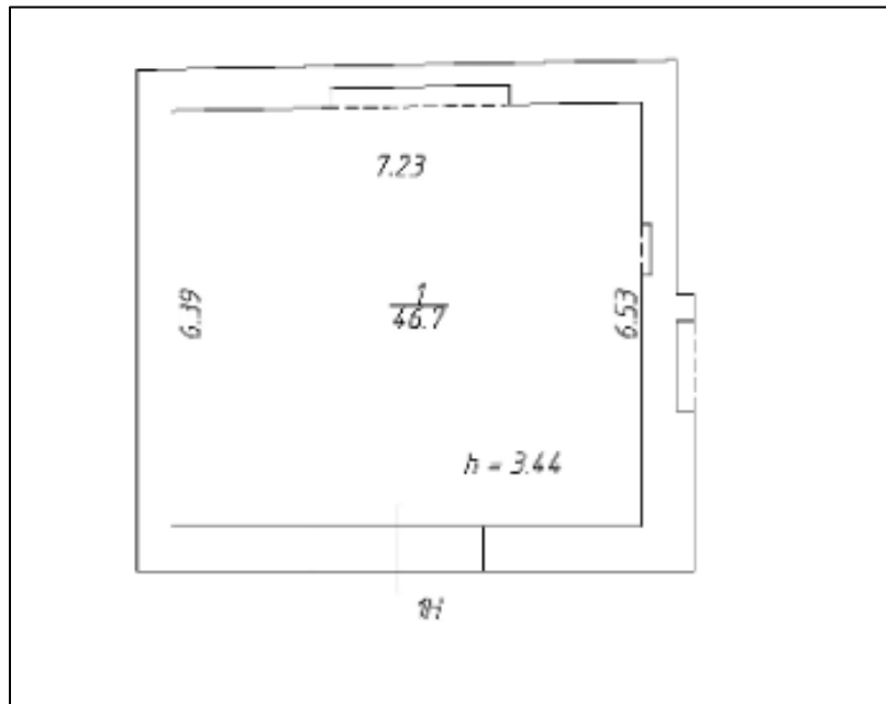
Рисунок 5. План здания
