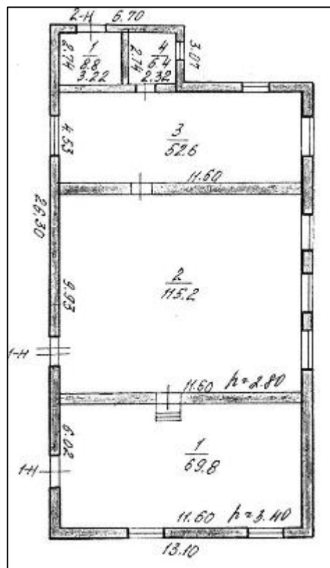
Рисунок 19. План 1 этажа здания литера К
