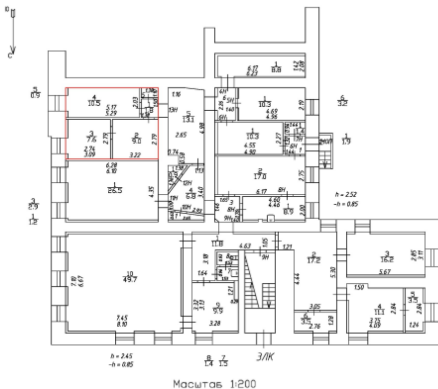
Фрагмент плана цокольного этажа, ЗЛК
