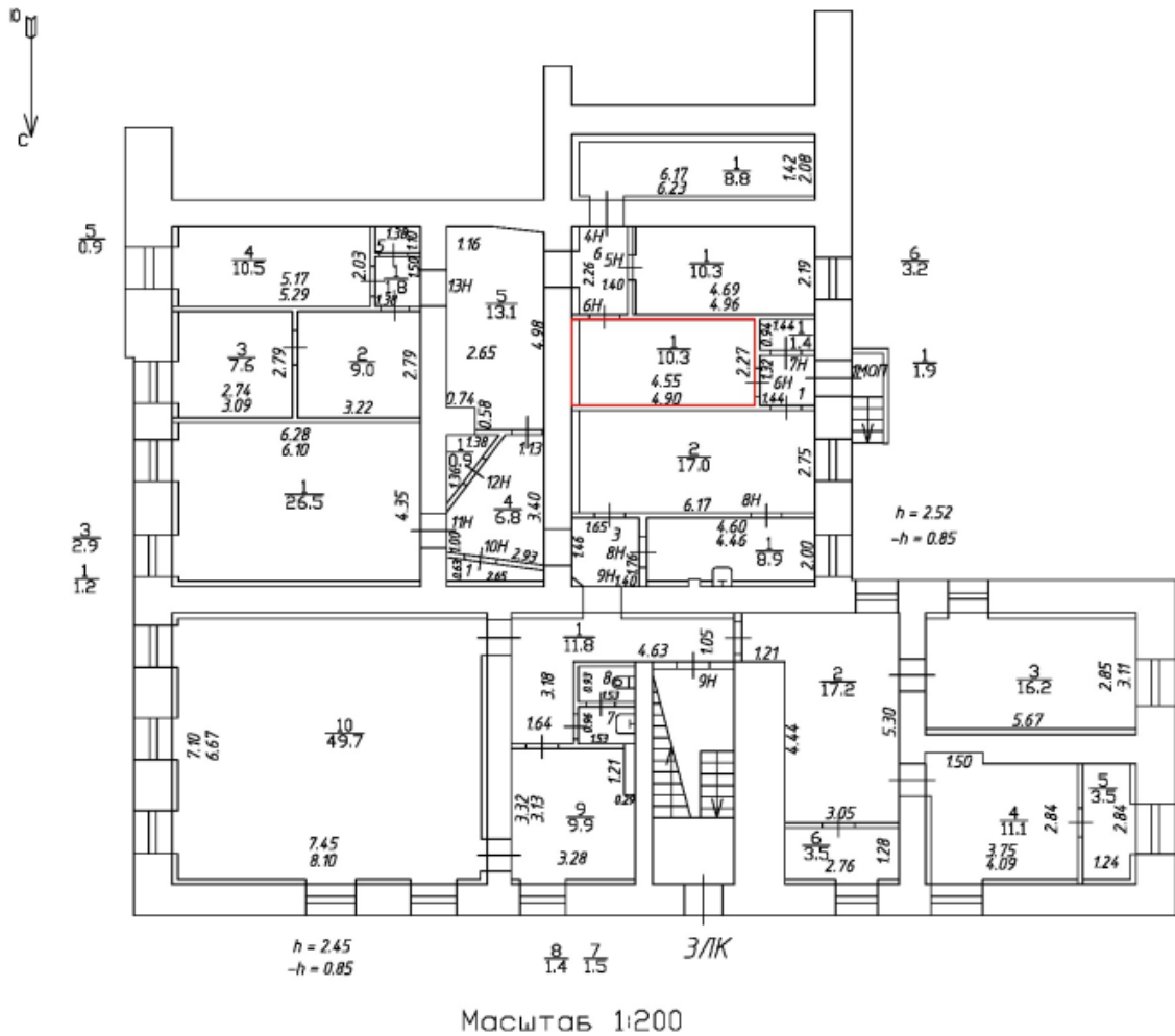
Фрагмент плана цокольного этажа, ЗЛК
