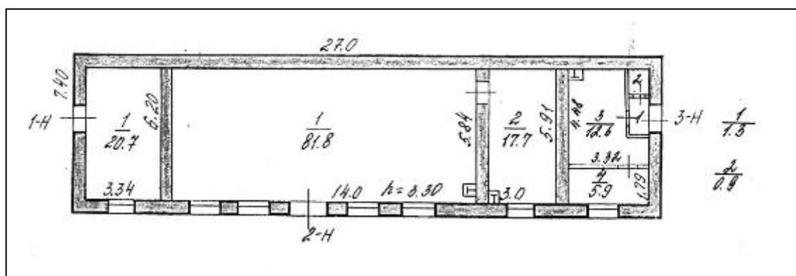
Рисунок 18. План 1 этажа здания литера З
