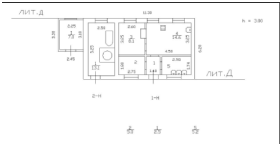
Рисунок 14. План 1 этаж литера Д
