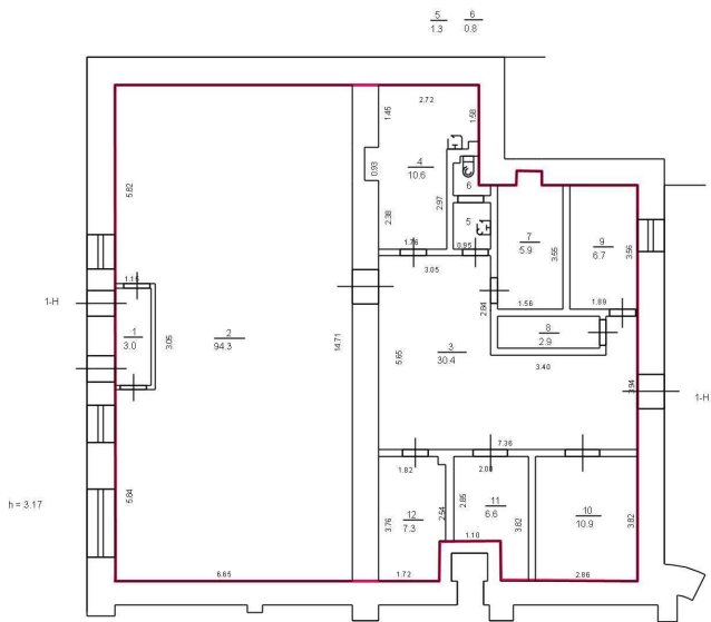
План части 1 этажа
