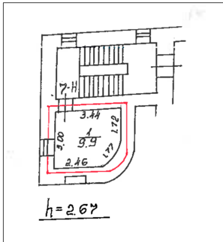
Рисунок 5. План оцениваемого помещения 7-Н
