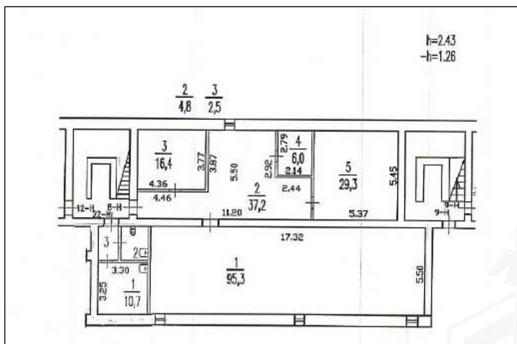
Рисунок 4. Расположение объекта на плане этажа
