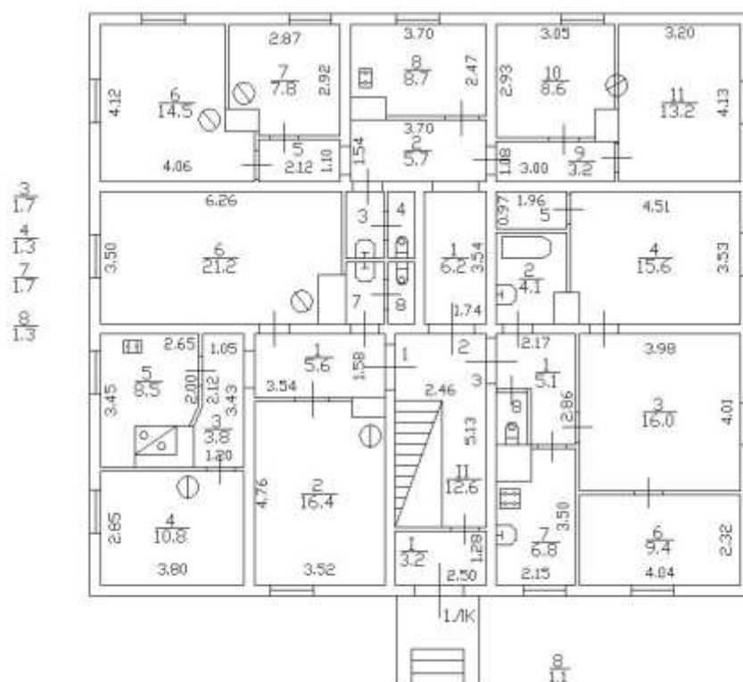
Рисунок 5. План 1 этажа
