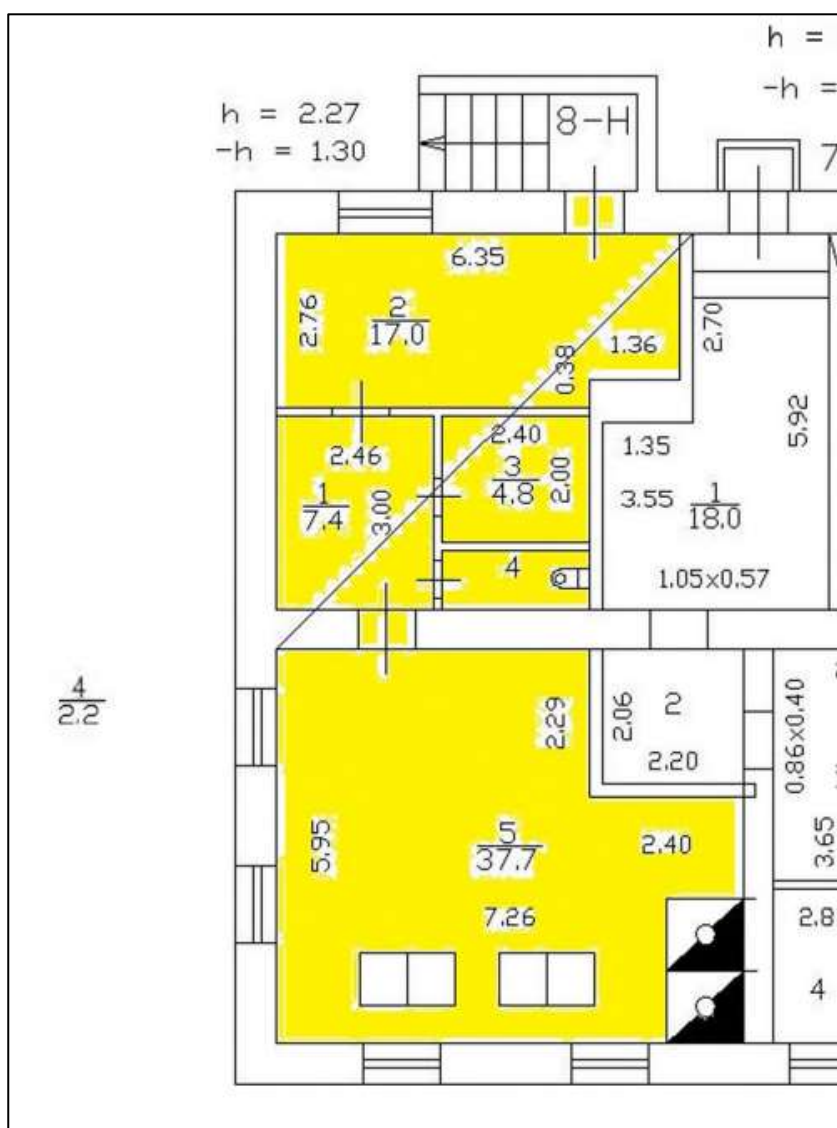
Рисунок 5. План оцениваемого помещения
