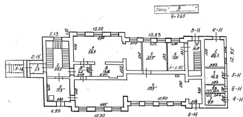
План 1 этажа
