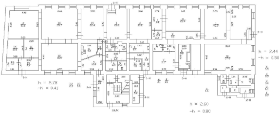
План 1 и цокольного этажа
