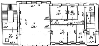
План 2 этажа
