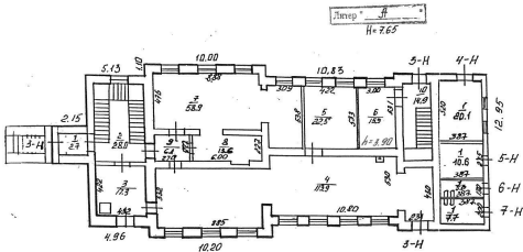
План 1 этажа
