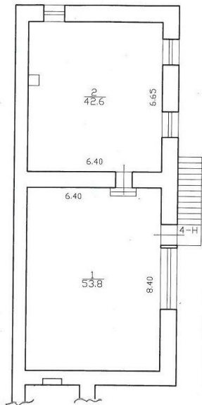
План 2 этажа
