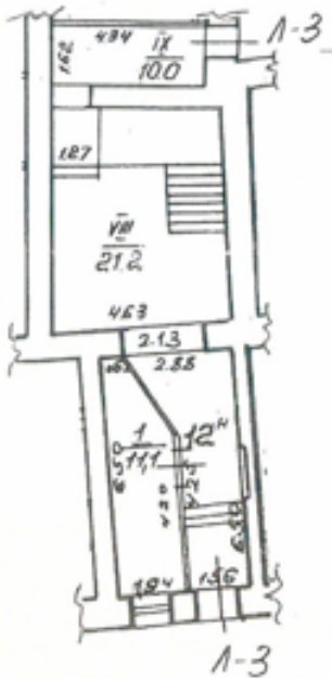
План 1 этажа
